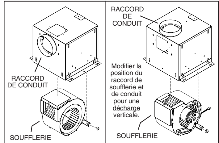
Raccord de soufflerie et de conduit en position de décharge horizontale (préassemblée)
